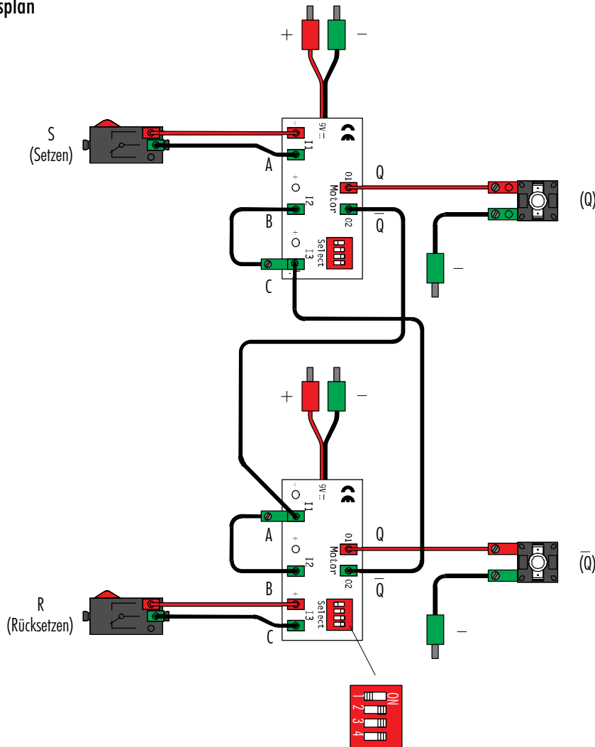
Schaltbild
